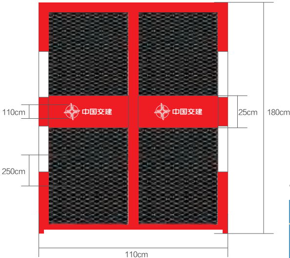
层站防护门
